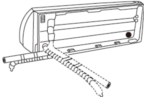
Kondenswasserschlauchanschluß rechts
