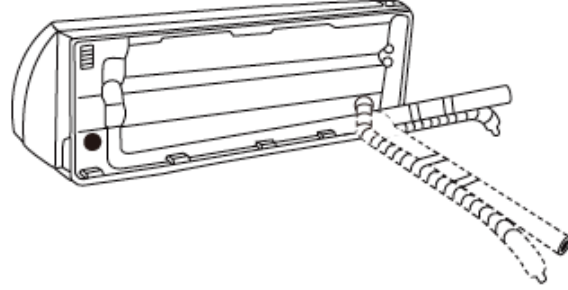
Kondenswasserschlauchanschluß links
